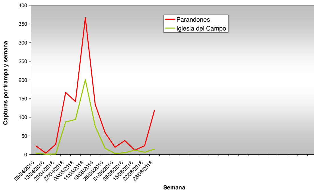
Curva de vuelo de Polilla del Racimo ( Lobesia botrana ) 2016
